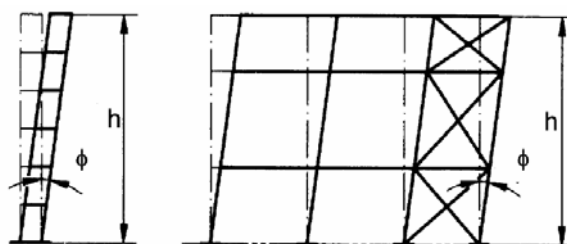
Figura C4.2.2 Imperfezioni globali equivalenti
