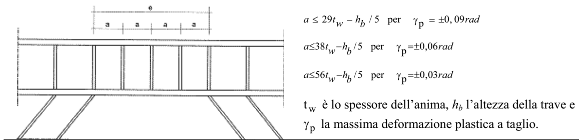
a) «Elementi di connessione corti»
