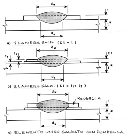
Figura C4.2.35 – Saldature a bottonne
