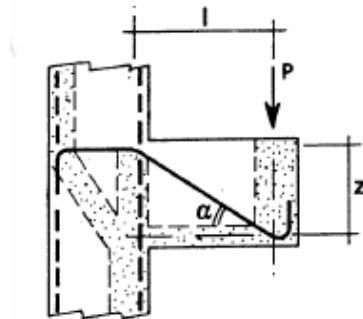
Figura C4.1.8 Esempi di modello a puntoni e tiranti con tirante obliquo per mensole tozze
