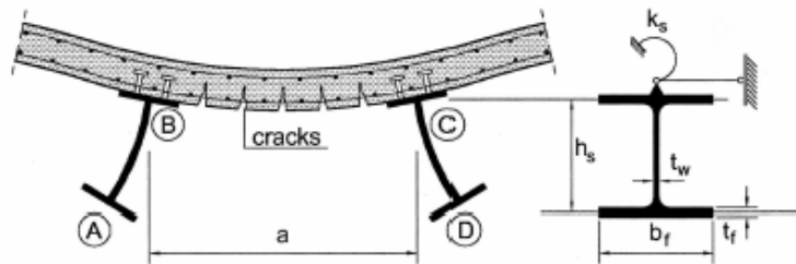
Figura C4.3.4. Telaio ad U invertita: A-B-C-D
