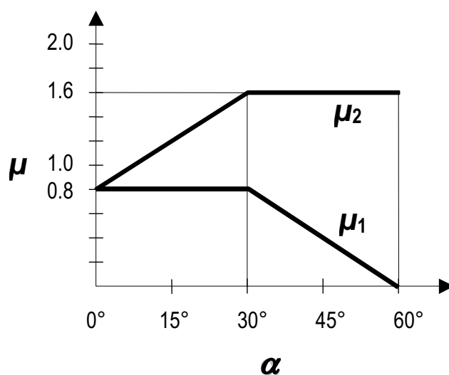
Figura C3.4.1: Coefficienti di forma per il carico neve
