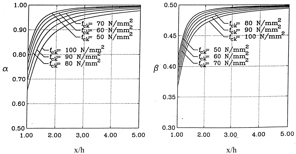
Fig. 4.6 - Valori dei coefficienti \alpha (di “riempimento”) e \beta (di “posizione”) per la regione 5.
