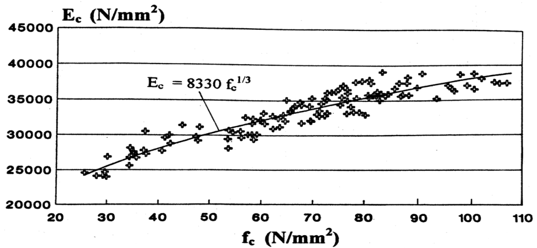
Fig. 4.4 - Risultati sperimentali e correlazione fra modulo elastico secante ( E_c ) e resistenza cilindrica a compressione, per calcestruzzi con aggregato a base di granito [4.3].
