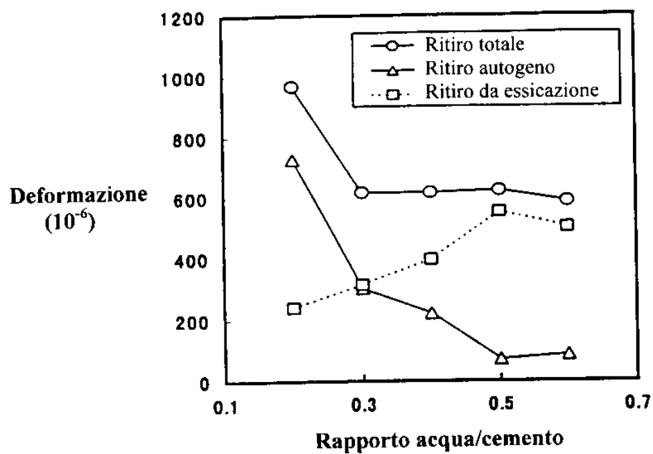
Fig. 7.4 - Varie forme di ritiro nel calcestruzzo [4.5]: totale, autogeno e da essiccazione, in funzione del rapporto a/c.
