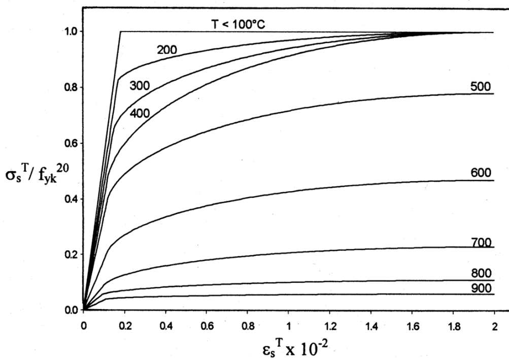
Fig. 2.5 – Diagrammi sforzo-deformazione per acciai da c.a. laminati a caldo, secondo il Bollettino CEB n. 174 [5.1].
