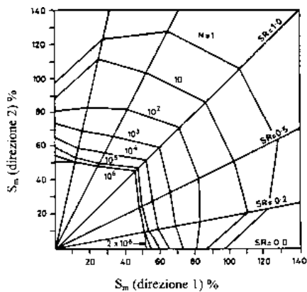
Fig. 3.3 - Comportamento a fatica di calcestruzzi soggetti a carichi ciclici alternati di trazione e compressione, a confronto col comportamento sotto carichi ciclici di sola compressione [3.4]: (a) f_c = 35 \text{ N/mm}^2 , e (b) f_c = 95 \text{ N/mm}^2 .
