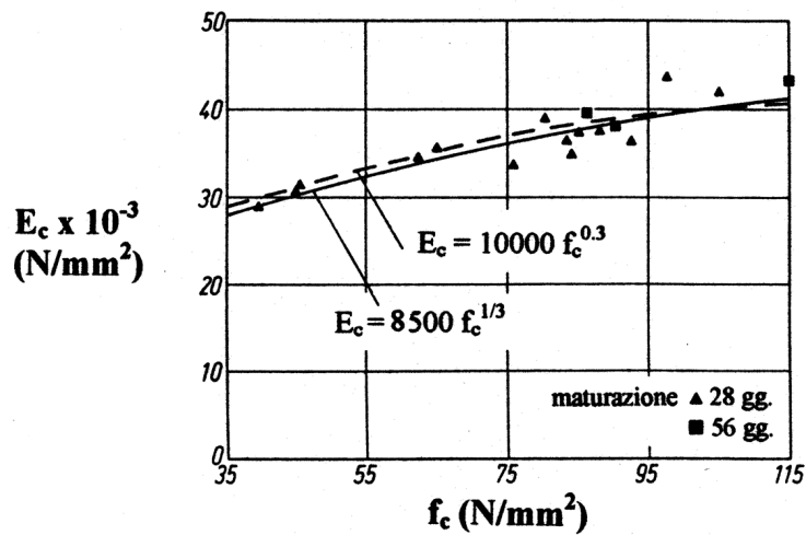
Fig. 5.4 - Correlazioni fra modulo elastico secante e resistenza cilindrica in compressione [1.2, 1.4, 4.1].
