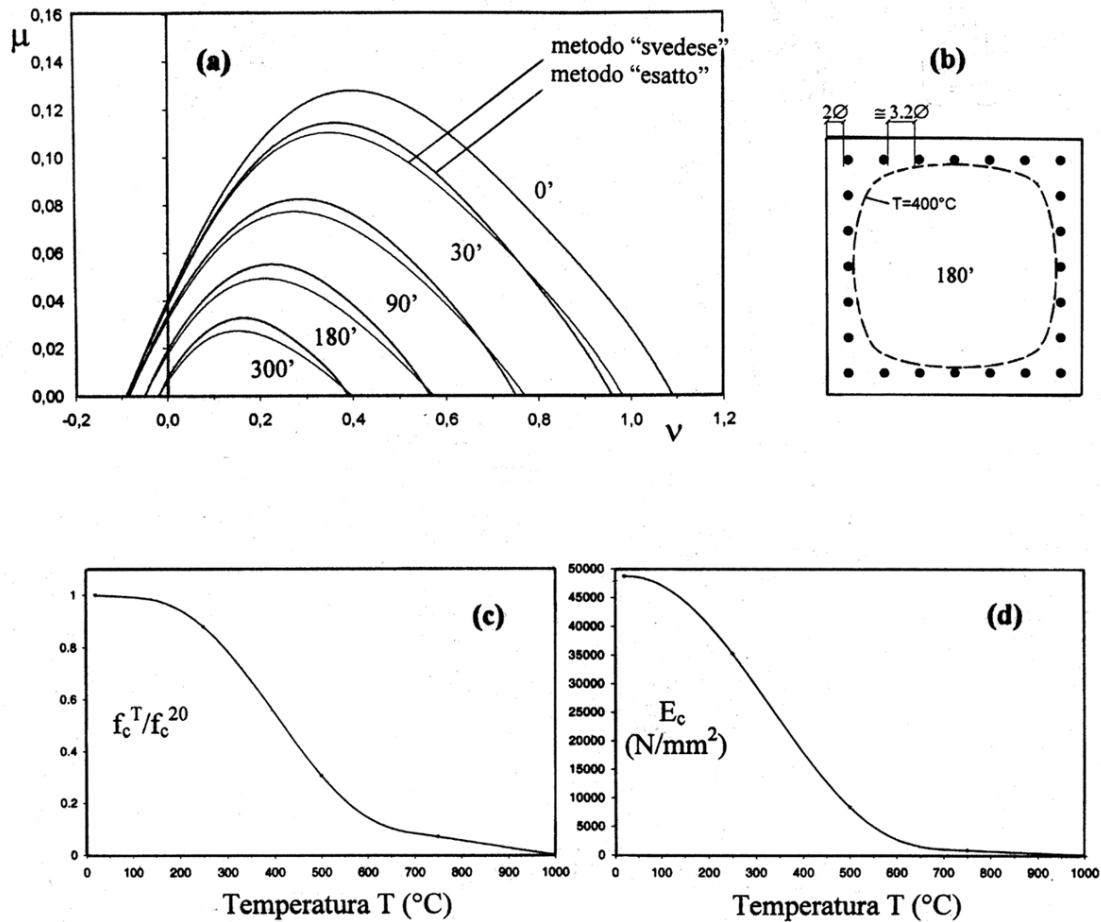
Fig. 3.5 – (a) Domini M-N per sezione quadrata di lato 60 cm, con percentuale d’armatura del 2%, soggetta ad incendio standard: simulazione numerica “esatta” (con le effettive caratteristiche a caldo del calcestruzzo) e previsione secondo il metodo di Anderberg (“svedese”) basato sull’isoterma 400^\circ\text{C} , con i domini adimensionalizzati rispetto a f_{ck}^T e f_{yk}^T . (b) Sezione 60 \times 60 cmq armata con 24 barre \varnothing 20 ; f_{ck}^{20} = 100 \text{ N/mm}^2 ; acciaio FeB44k. (c,d) Curve resistenza a compressione - temperatura e modulo elastico secante - temperatura adottate nell’analisi [5.9]
