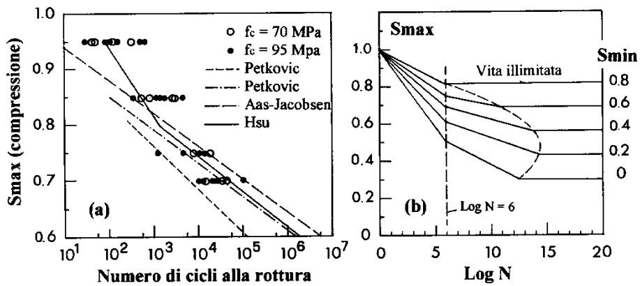
Fig. 2.3 - (a) Curve S-N in compressione, e risultati sperimentali [3.4]; e (b) proposta per calcestruzzi ad alte prestazioni (Petkovic et al. [1.3]): \log N = k (12 + 16 S_{\min} + 8 S_{\min}^2) (1 - S_{\max}) ove k = 1 per \log N \leq 6 , e k = 1 + 0.2 (\log N - 6) per \log N > 6 .
