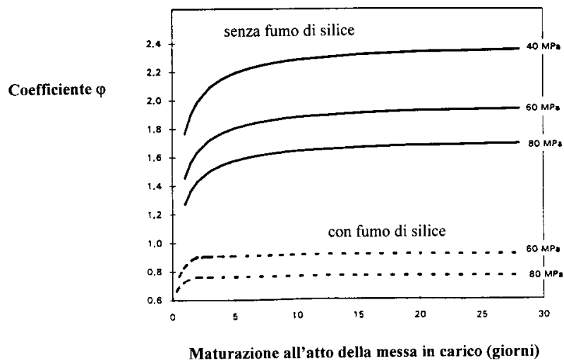
Fig. 11.4 – Diagrammi del coefficiente di viscosità per calcestruzzo NR e AR, con e senza fumo di silice [4.2].
