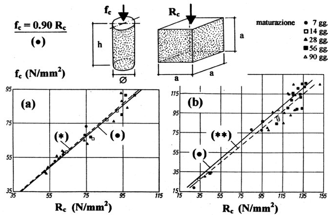
Fig. 1.4 - Correlazione fra resistenza cilindrica e cubica [4.1]: (a) \varnothing = 150 , h = 300 , a = 200 mm; e (b) \varnothing = 100 , h = 200 , a = 100 mm. (*) e (**) = regressioni lineari.
