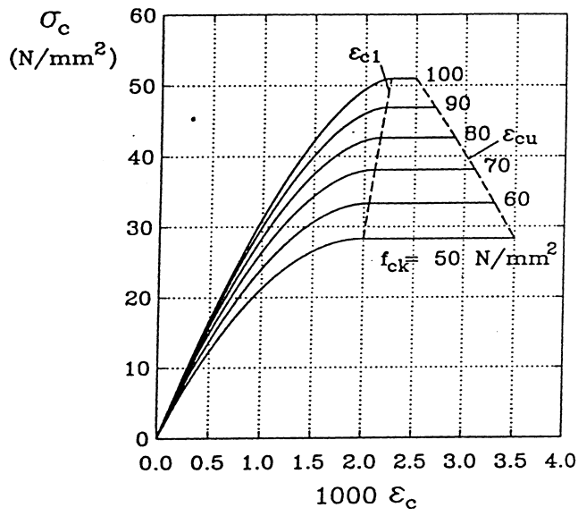
Fig. 1.6 - Diagrammi \sigma_c - \epsilon_c per calcestruzzi ad alte prestazioni/alta resistenza.
