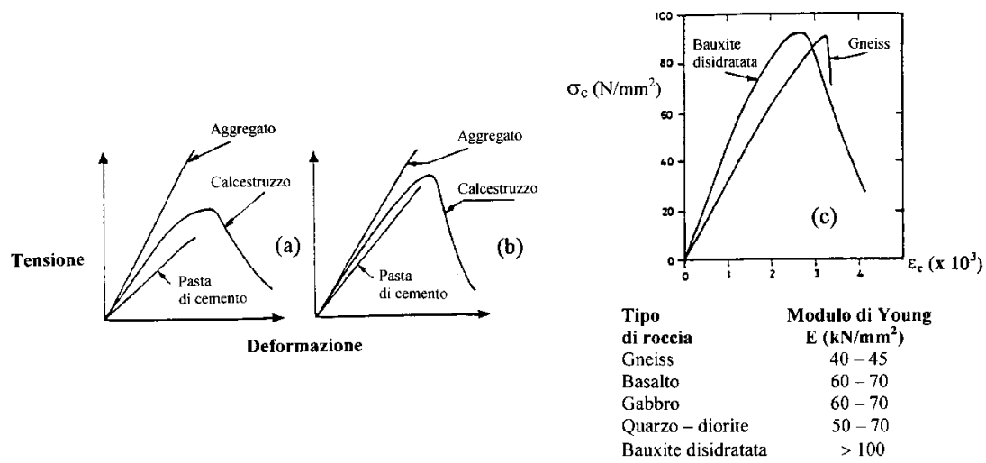
Fig. 3.2 - Influenza della resistenza dell'aggregato e della pasta cementizia sul comportamento costitutivo di un calcestruzzo NR (a) e AR (b), e sul modulo elastico (c) [1.3].
