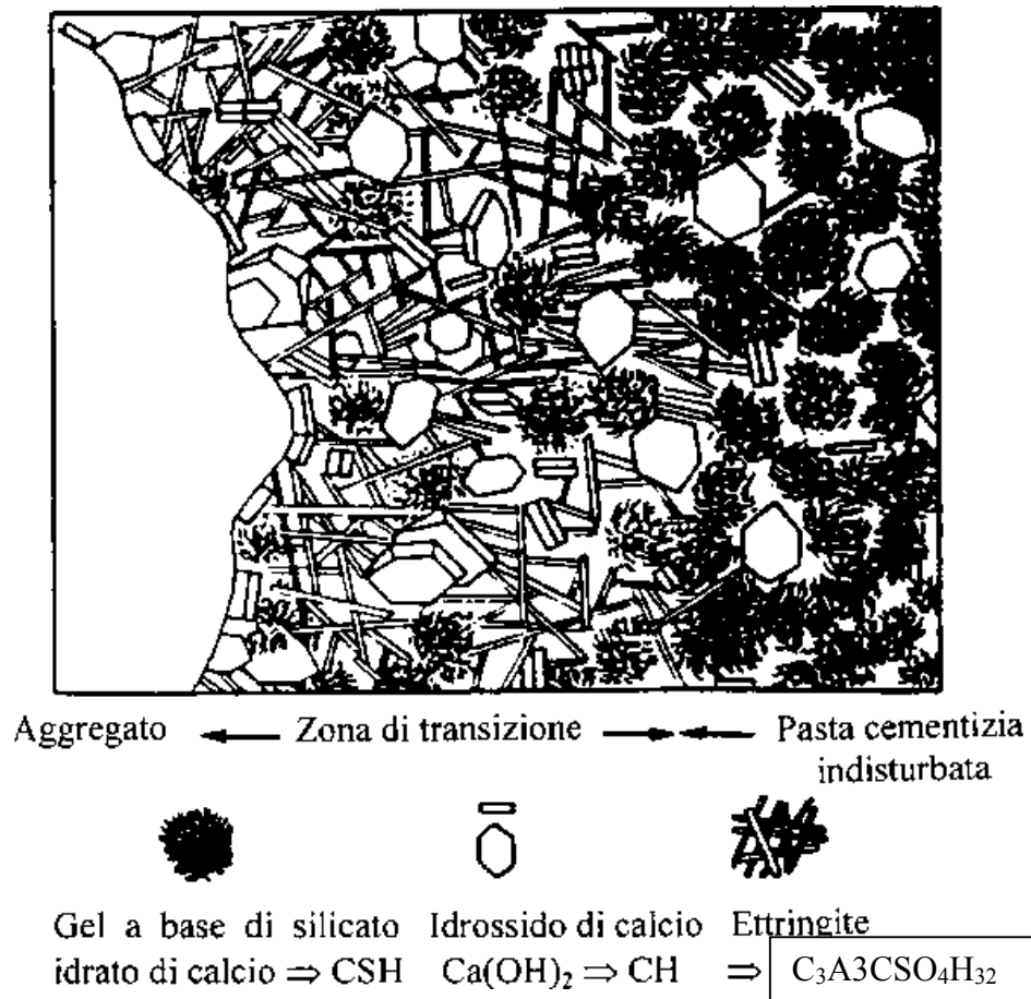
Fig. 1.2 - Zona di transizione all'interfaccia pasta cementizia-aggregato [1.2].
