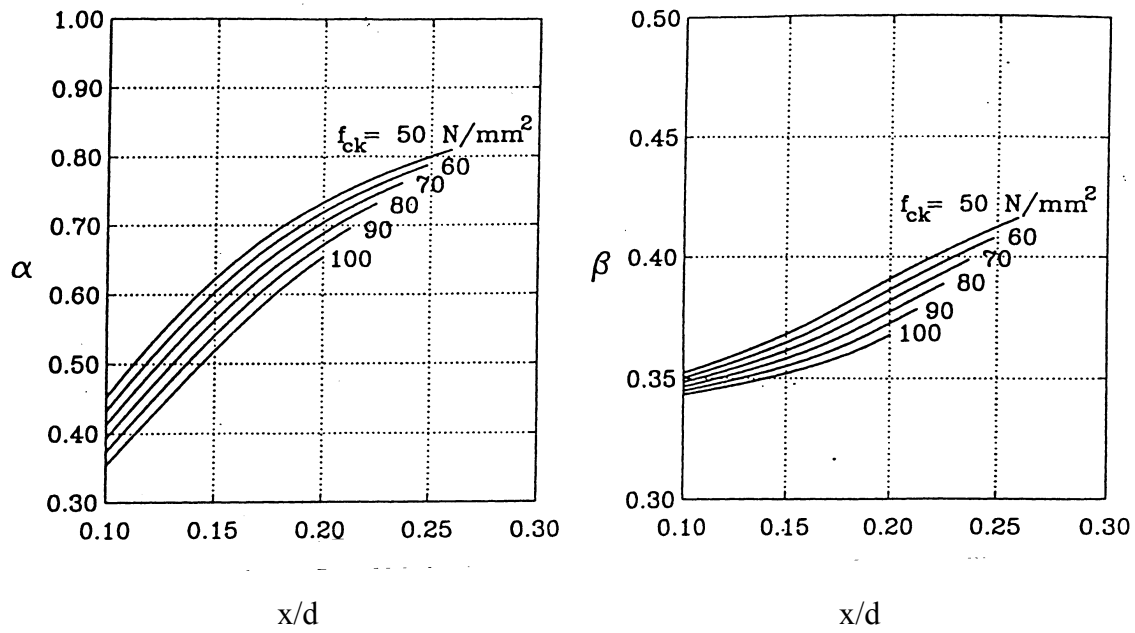
Fig. 3.6 - Valori dei coefficienti \alpha (di “riempimento”) e \beta (di “posizione”) per le regioni 2-3-4.
