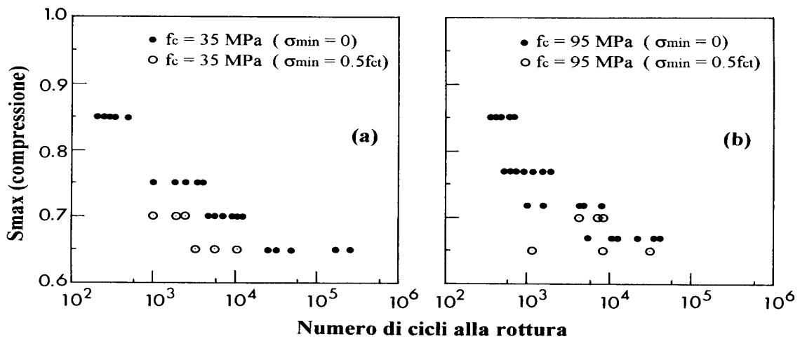
Fig. 3.3 - Comportamento a fatica di calcestruzzi soggetti a carichi ciclici alternati di trazione e compressione, a confronto col comportamento sotto carichi ciclici di sola compressione [3.4]: (a) f_c = 35 \text{ N/mm}^2 , e (b) f_c = 95 \text{ N/mm}^2 .
