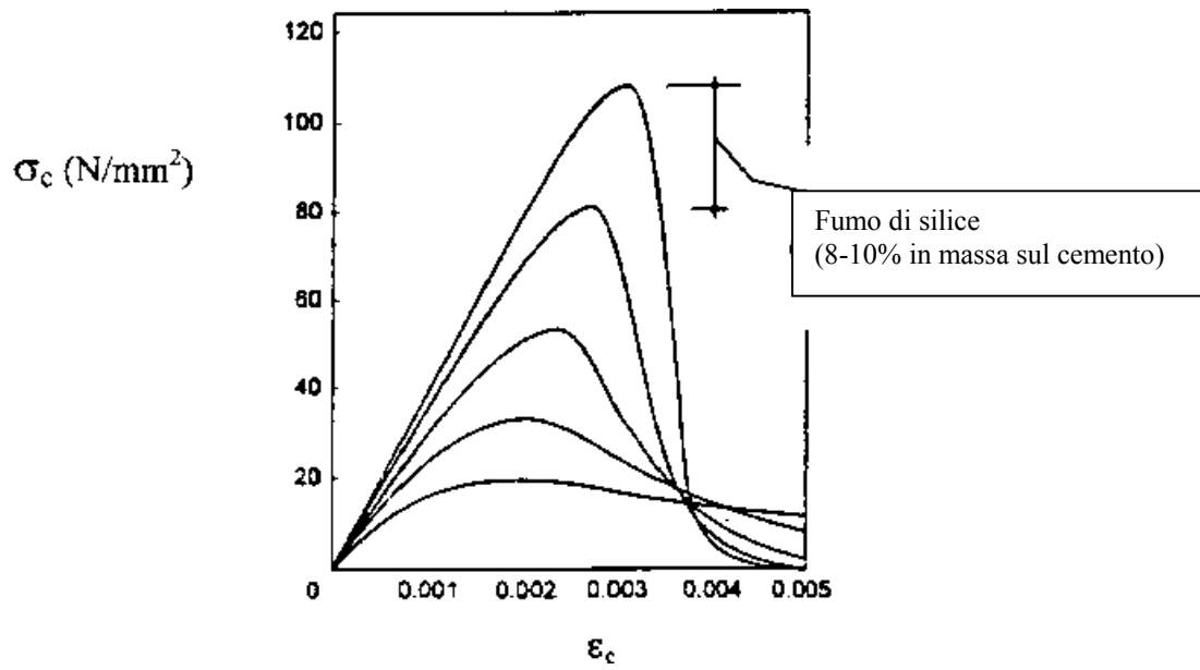
Fig. 2.2 - Effetti dell'introduzione del fumo di silice per ottenere resistenze a compressione superiori a 80 N/mm 2 [1.3].
