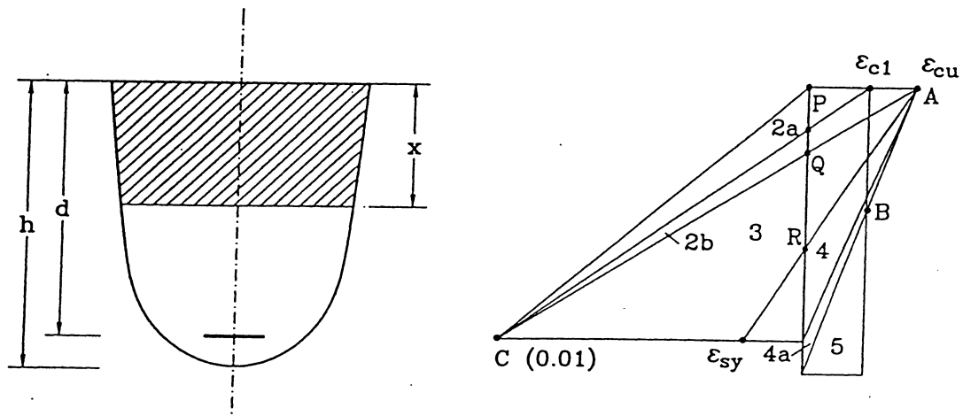
Fig. 2.6 - Frontiere delle regioni di verifica.
