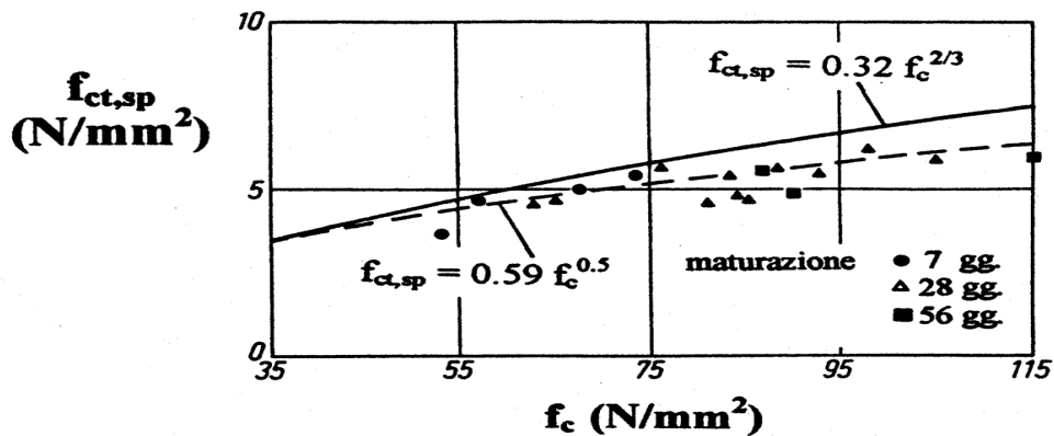
Fig. 3.4 - Correlazioni fra resistenza a trazione indiretta per spacco ( f_{ct,sp} ) e resistenza cilindrica in compressione [4.2].
