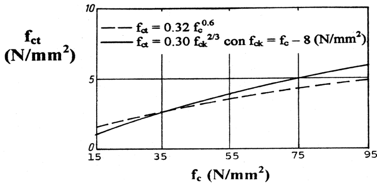
Fig. 2.4 - Correlazioni fra resistenza a trazione diretta e resistenza cilindrica in compressione [4.1].
