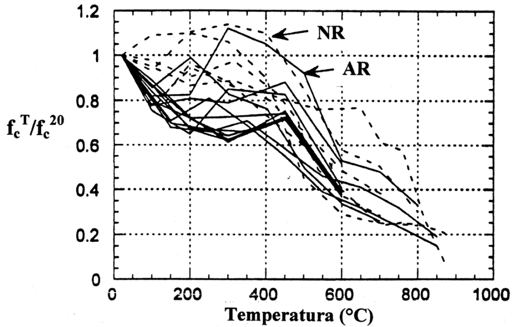
Fig. 1.5 – Diagrammi della resistenza a compressione di calcestruzzi normali (NR) e ad alta resistenza (AR) in funzione della temperatura, in rapporto alla resistenza a temperatura ambiente (20°C) [5.3]. Provini scarichi durante il riscaldamento.
